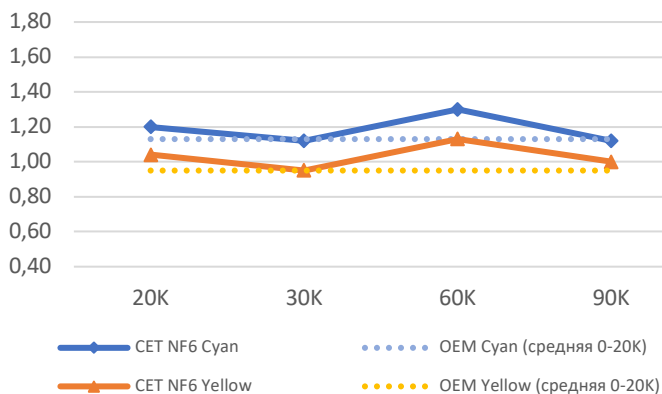
Плотность печати за длительный период, Cyan и Yellow
