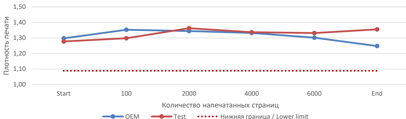
ECOSYS M2040dn
